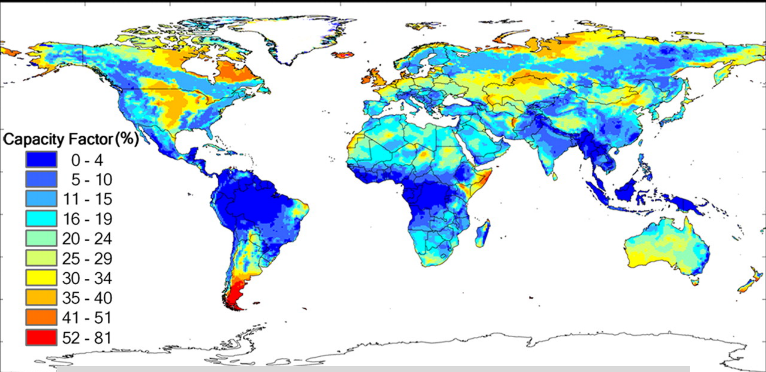
Мировое распределение коэффициента ветроемкости на суше (%) на высоте 100 м (Lu et al. 2009) Global distribution of onshore capacity factor (%) for winds at 100 m (Lu et al. 2009)
